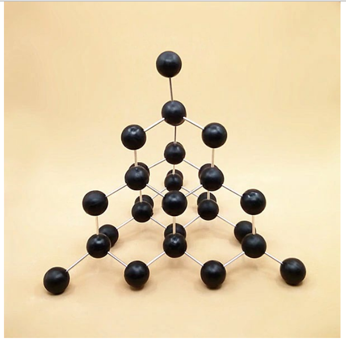
kryštalová štruktúra
